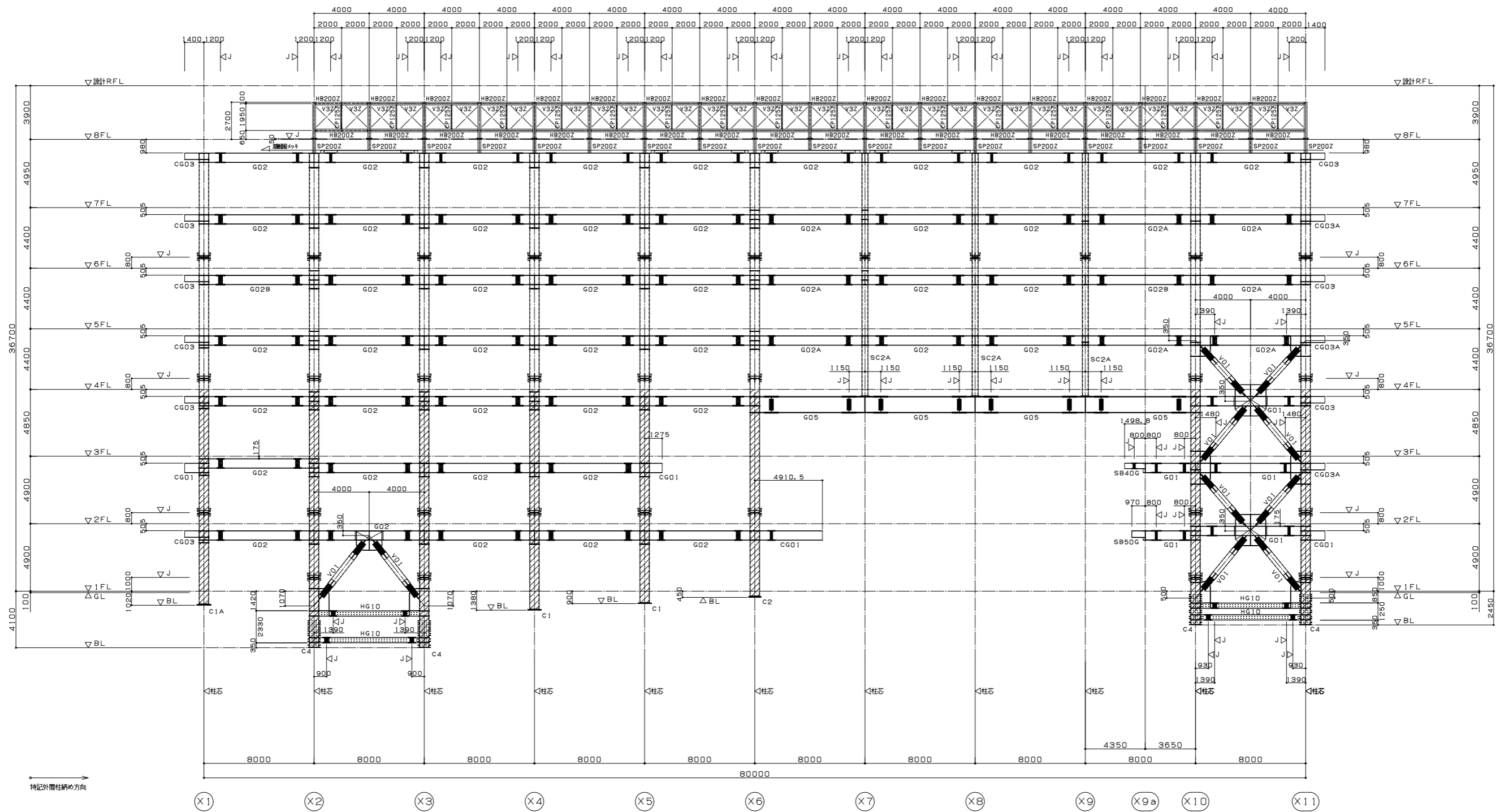
Y3通り軸組図 1/150 斜線部は、CFT柱とする
