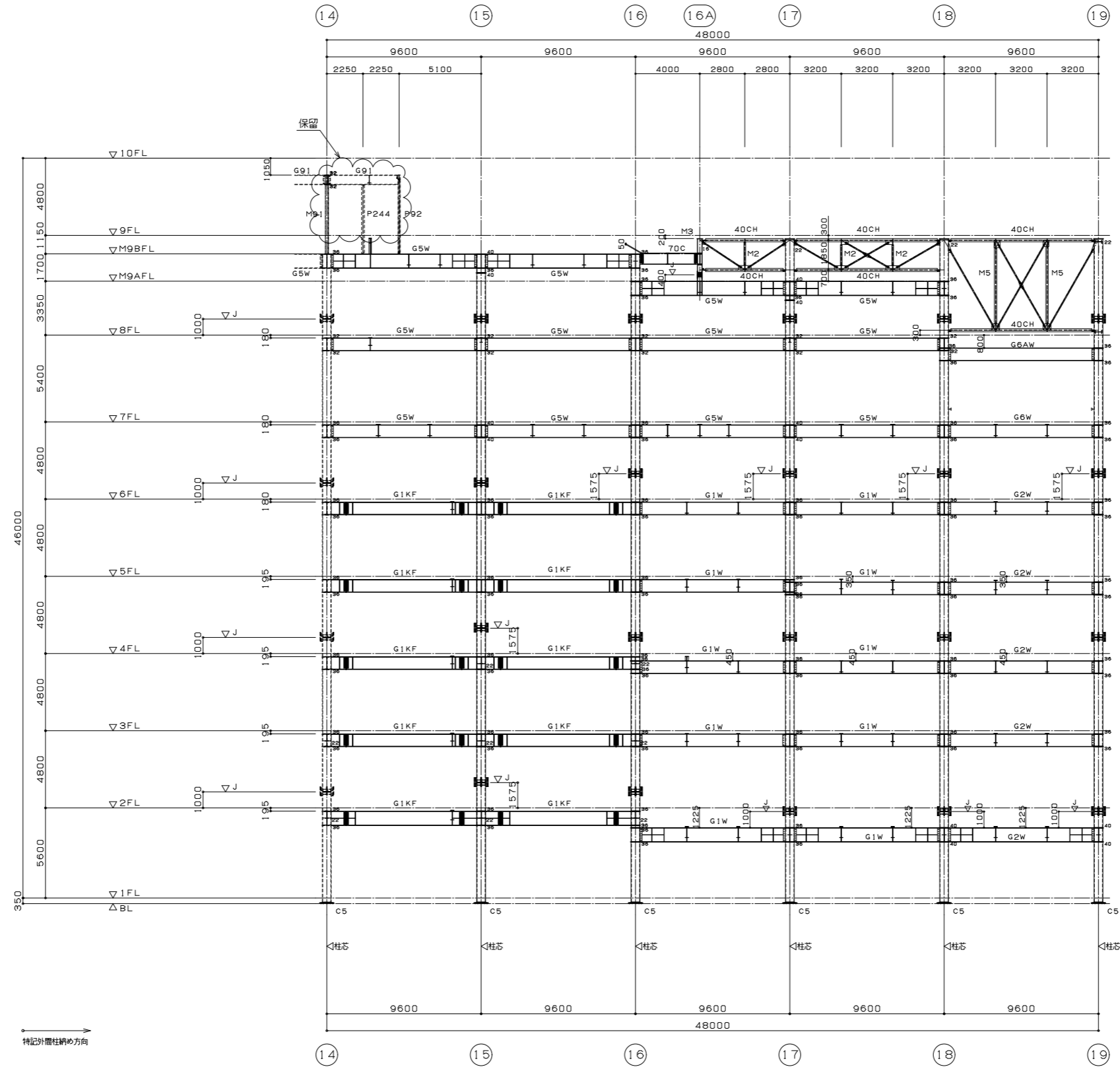
A通り軸組図 1/150 特記無き 軸ブレースは ZV11 とする
