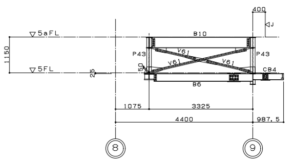
C通り-1100 軸組図
